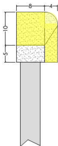
Profilato ad U in alluminio 60x20 - 25 mm.
